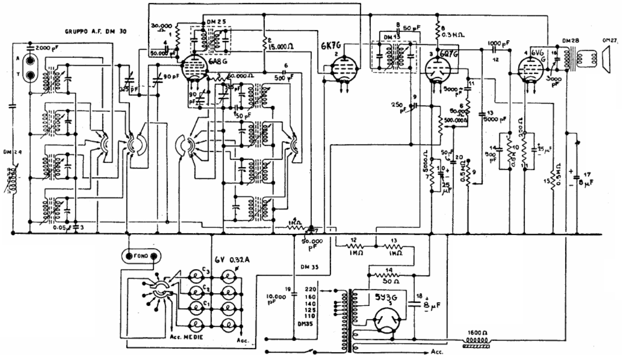
IMER RADIO - Mod. VERBANO - Onde medie da 190 a 580, corte da 32 a 52 m, da 20 a 32 m, da 12,5 a 20 m. MF: 467 kc/s. Potenza d'uscita circa 3,5 W.
